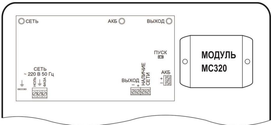
Рисунок 2 - общий вид без крышки
